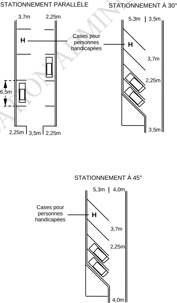
Dimensions relatives aux cases de stationnement, aux allées d'accès et aux allées de circulation
