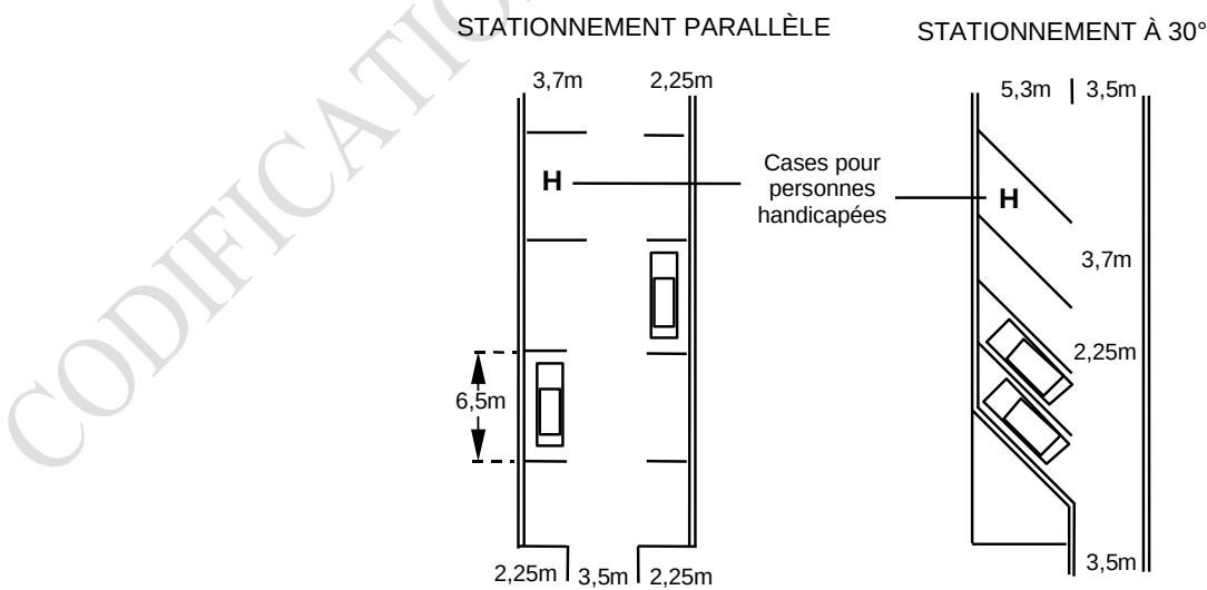
Dimensions relatives aux cases de stationnement, aux allées d'accès et aux allées de circulation
