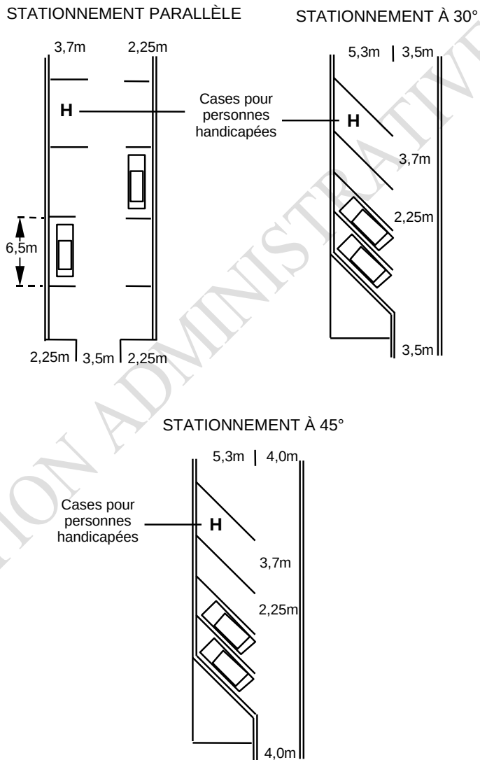
Dimensions relatives aux cases de stationnement aux allées d'accès et aux allées de circulation
